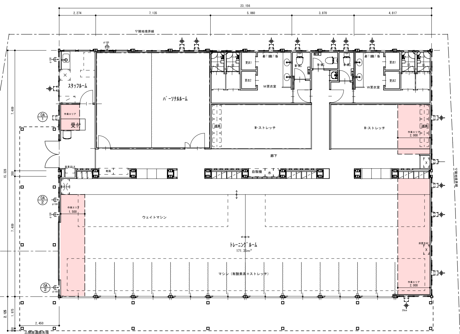
1階平面図
